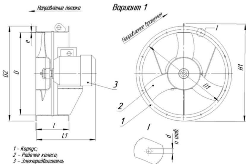
Рисунок 1 Габаритные и присоединительные размеры
