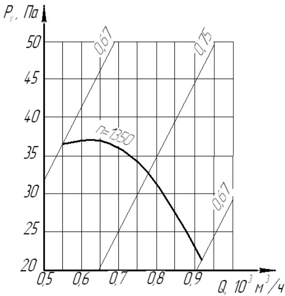
Рисунок 3 Аэродинамическая характеристика ВО-06-300-2,5
