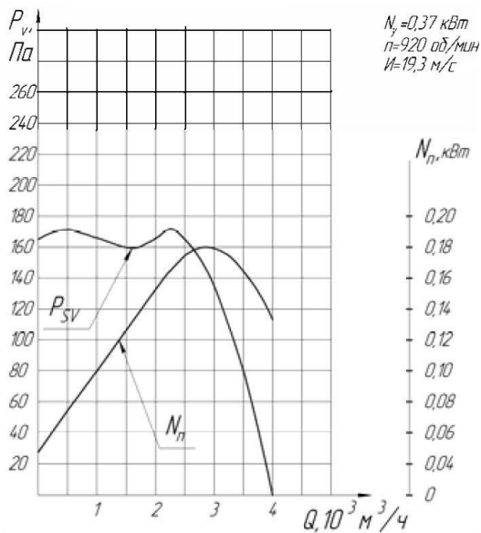
Рисунок 2 – Аэродинамические характеристики ВКР-4
