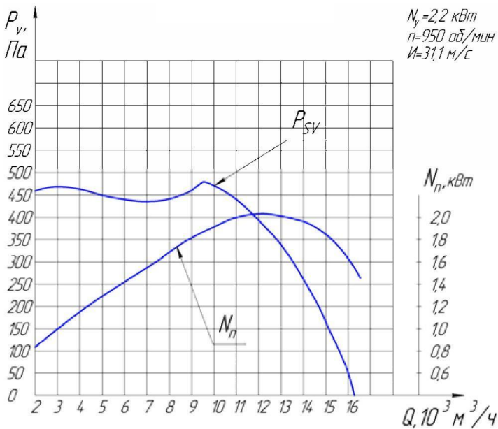
Рисунок 4— Аэродинамические характеристики ВКР-6,3
