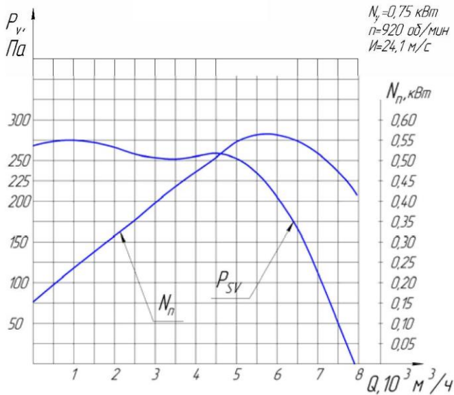
Рисунок 3 – Аэродинамические характеристики ВКР-5
