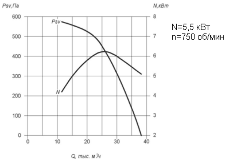
Рисунок 6– Аэродинамические характеристики ВКР-10
