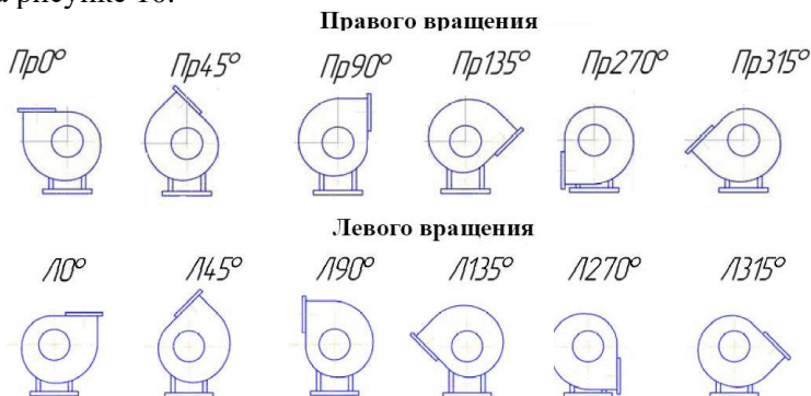
Рисунок 10 – Возможные положения корпуса вентилятора
