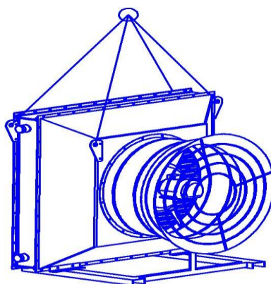
Схема строповки
